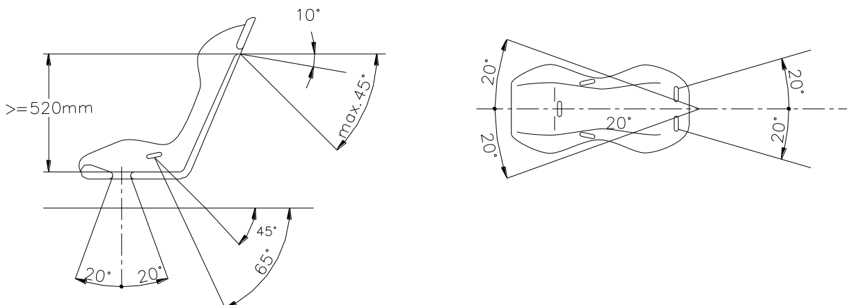
Zeichnung 253-61
