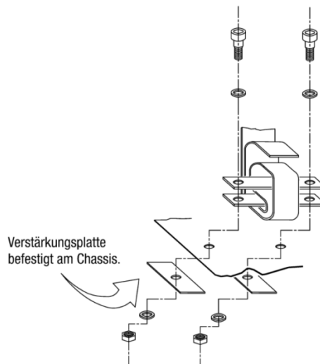
Zeichnung 253-64
