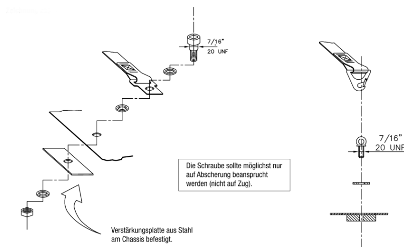
Zeichnung 253-62
