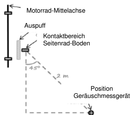
Sidecar - Draufsicht
