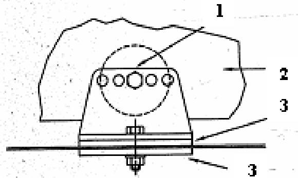
1 - Verstärkung 2 - Sitzschale 3 - Gegenplatte
