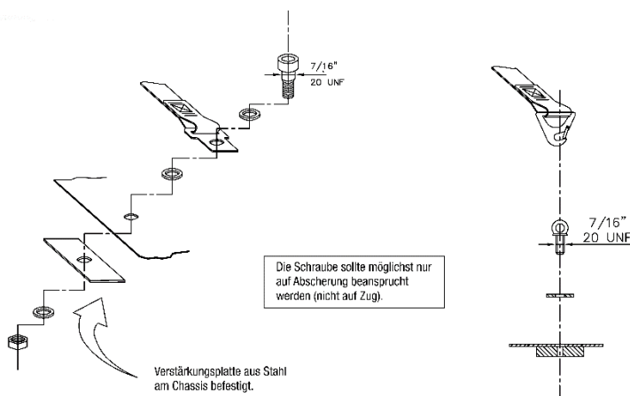
Zeichnung 2
