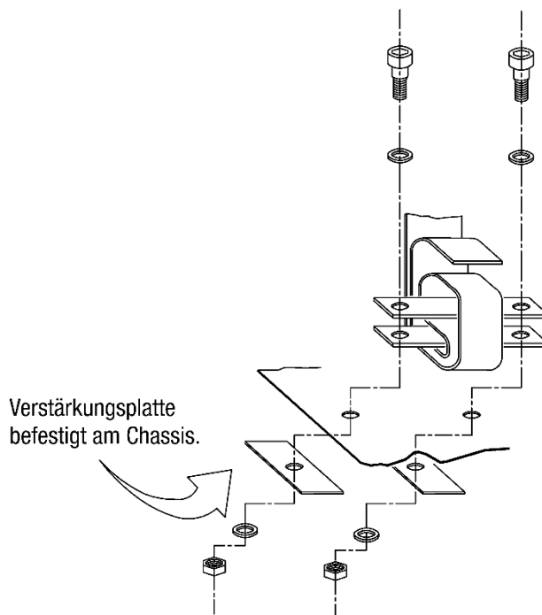
Zeichnung 4
